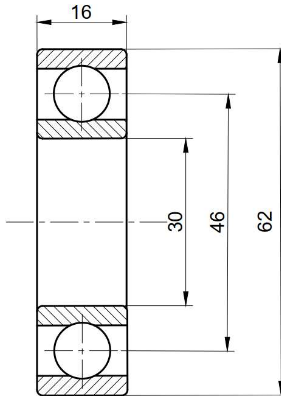
Potongan C-C
